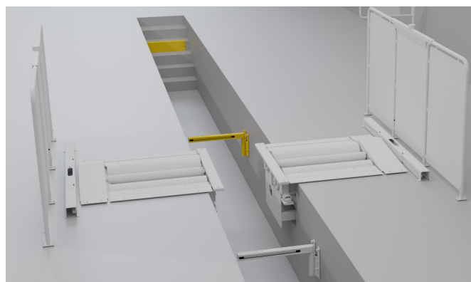
AM124124 KIT DE SÉCURITÉ BASSE - 1 portillon, 1 marche AM124125 KIT DE SÉCURITÉ BASSE - 2 marches (1 à l'entrée + 1 à la sortie de la fosse)
